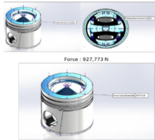
Fig. 3.7. Load position
